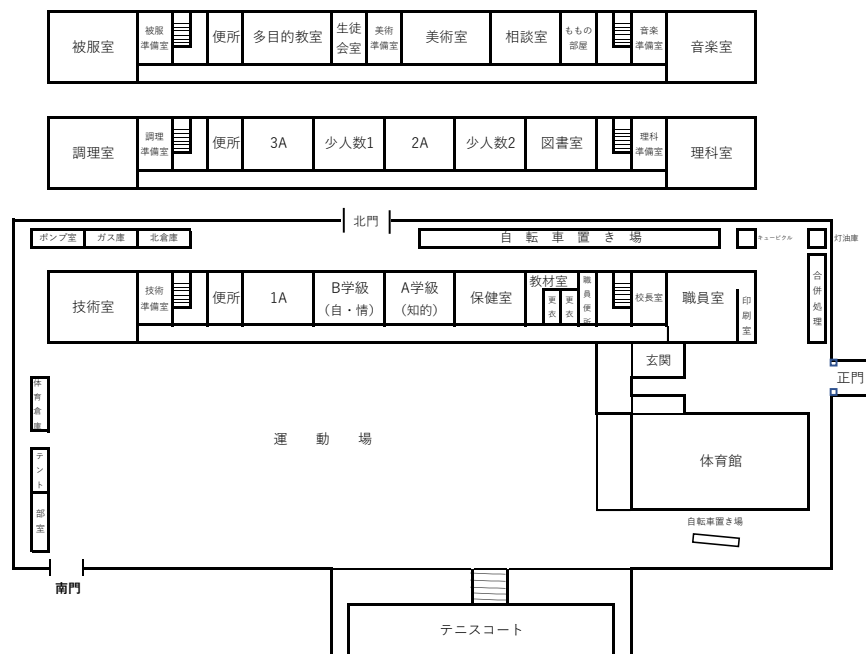
笠岡市・矢掛町中学校組合立小北中学校校舎配置図
